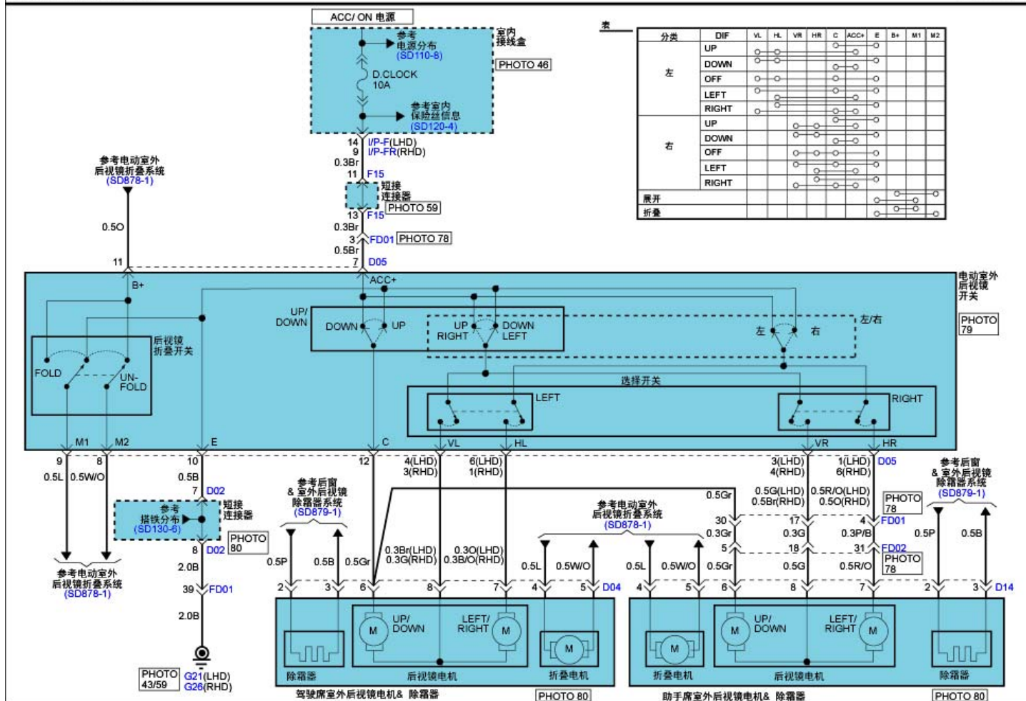
电动室外后视镜(1)
